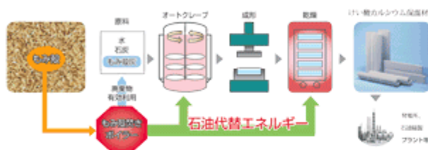
バイオマスを原材料及び燃料にしたけい酸カルシウム保温材の製造工程
