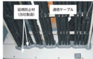
防火壁のケーブル貫通部の耐火工法
